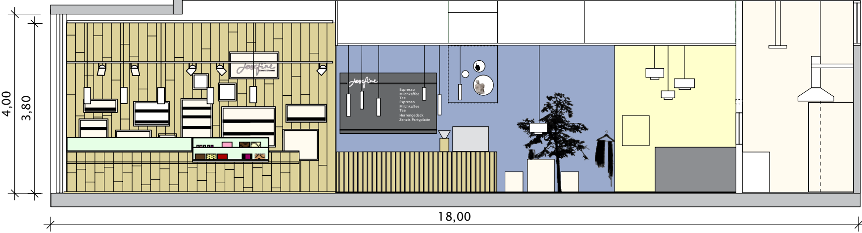
Südensicht
