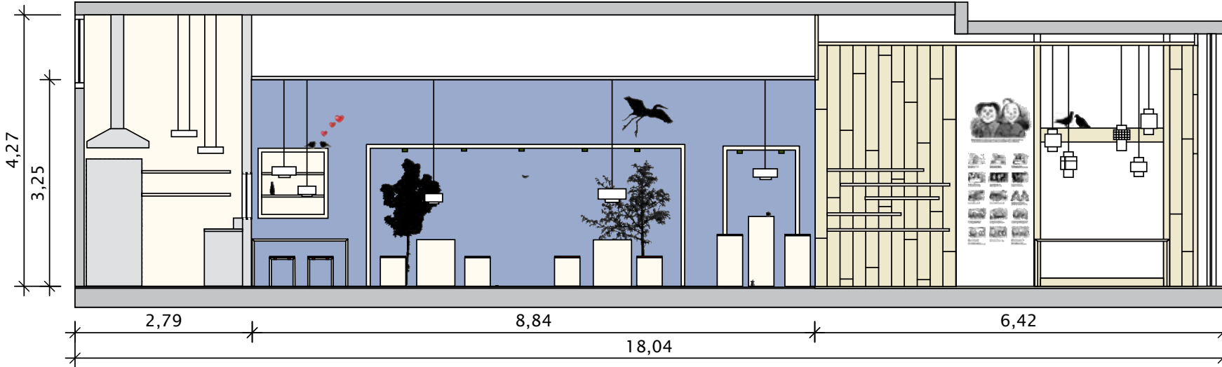
Nordansicht
